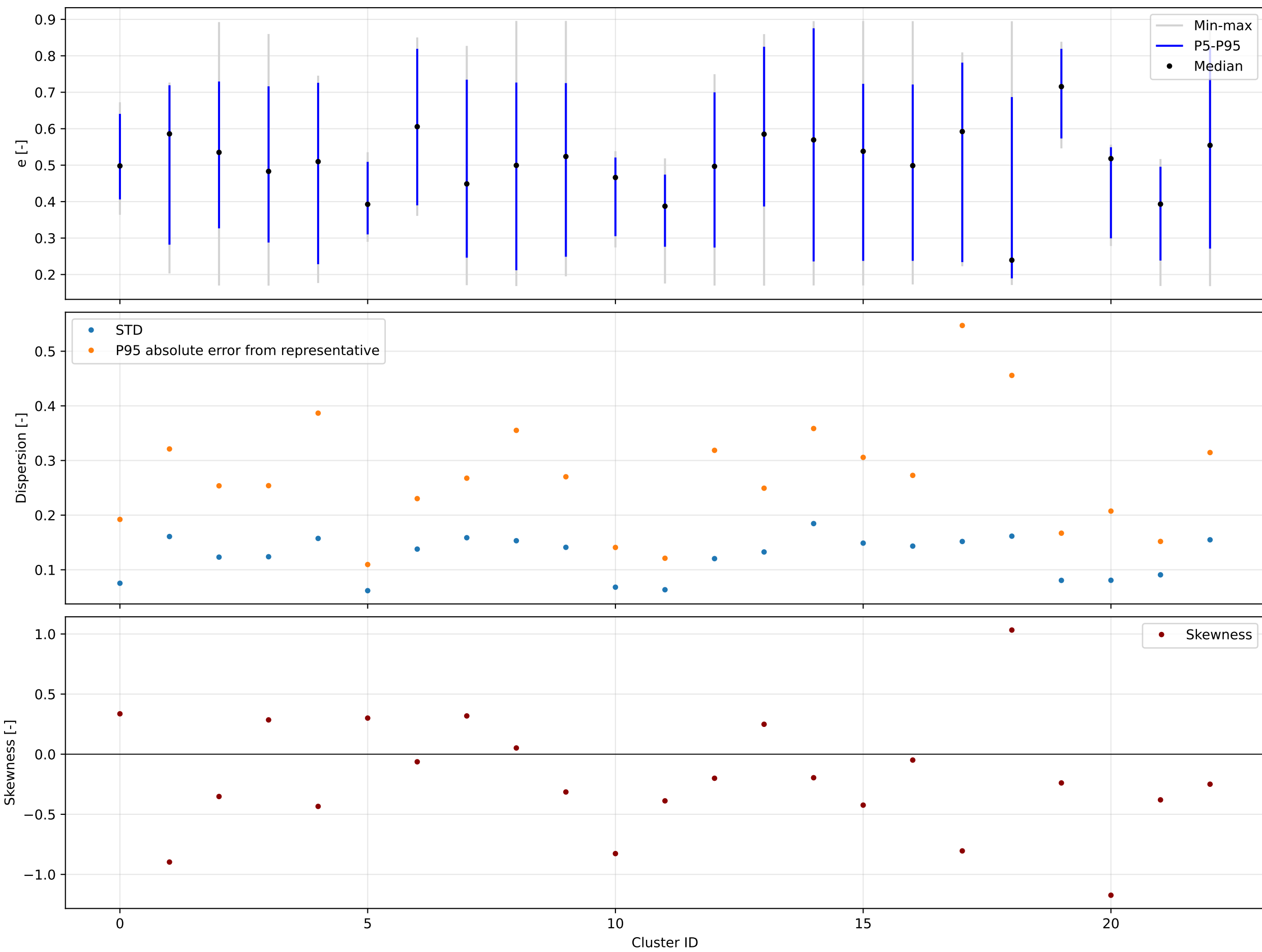
K=23 | backward | e | valid=194058/194058
